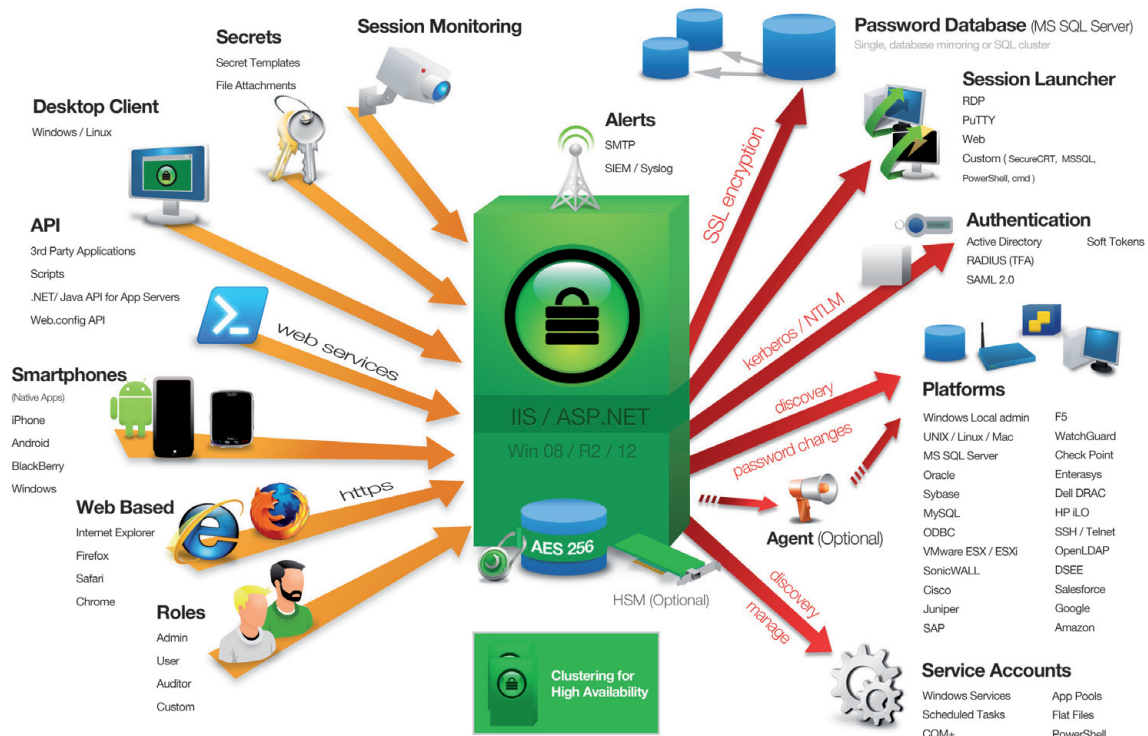
Obrázok 1: SECRET SERVER Architecture diagram
